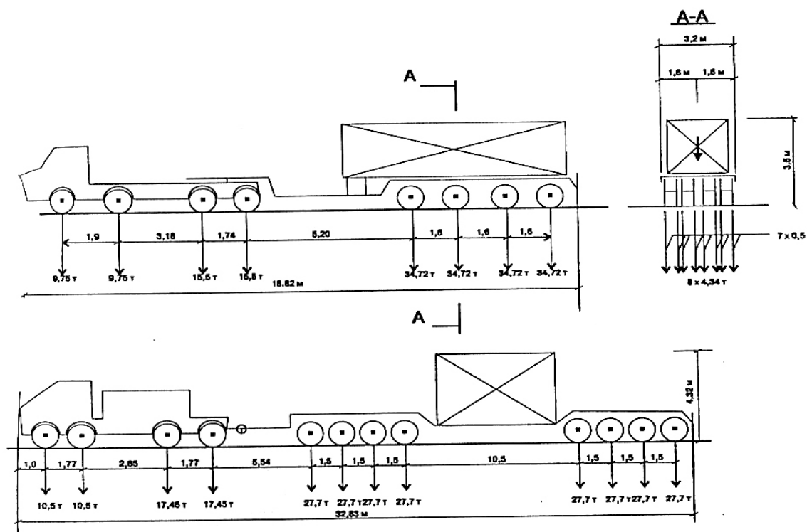
Примеры изображения схемы автопоезда
